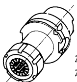
ER collet chuck 214-31737 (ER25M, H160) 214-31779 (ER25M, H150) 214-31708 (ER32, H100) 214-31780 (ER32, H90)
