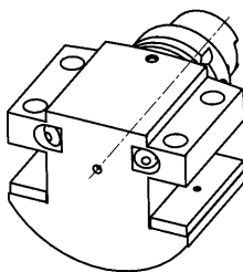
Axial toolholder 32x32/25x25 mm 142-11405
