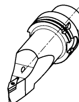
SVVCN H63ASVVCN16-L145
